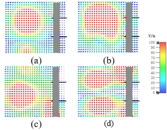
Fig. 4. The E-field distribution on the 1 m plane at 20.6 MHz (a) t=0 ; (b) t=T/4 ; at 24.2 MHz; (c) t=0 ; (d) t=T/4 .
